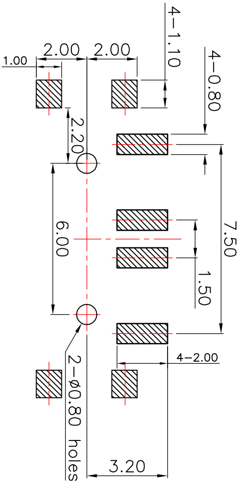
PCB Layout(Pattern side)
