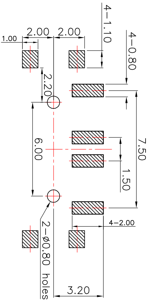
PCB Layout(Pattern side)
