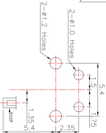
PCB Layout(Pattern side) Scale: 1 : 2
