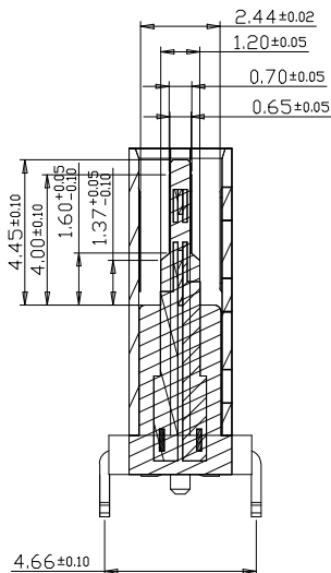
截面 1-1
