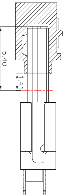
配合示意图
