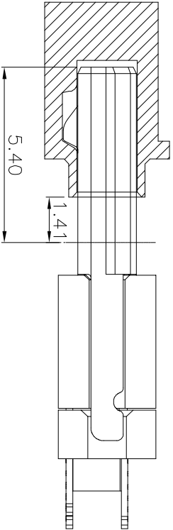
B-B 剖视图
