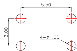
PCB Layout(Pattern Side)
