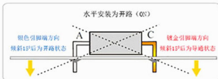
单方向倾斜15度触发型开关
