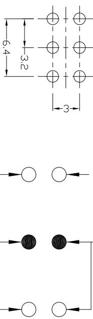
P.C.B LAYOUT
