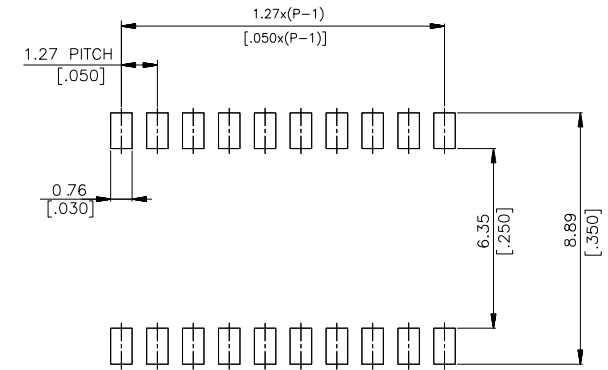
P.C.B. LAYOUT
